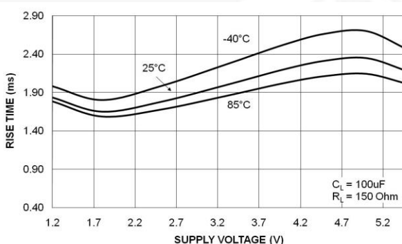
图 21. t_r 与电源电压的关系
