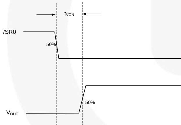
图 30. /SR0 上电
