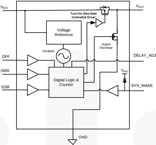
图 3. 框图
