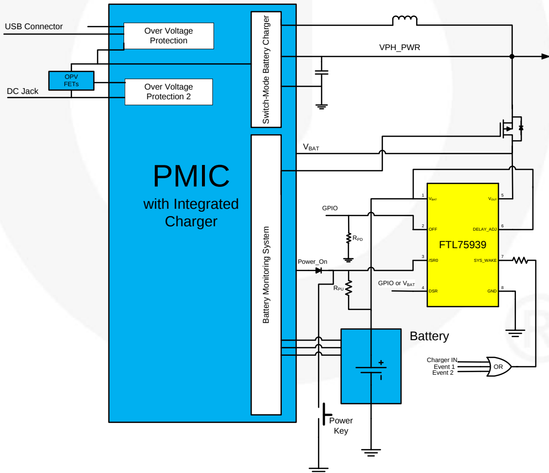
图 2. 带集成式充电器的典型应用 PMIC
