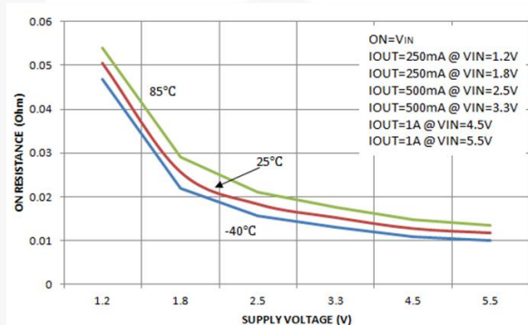
图 17. R_{ON} 与电源电压的关系
