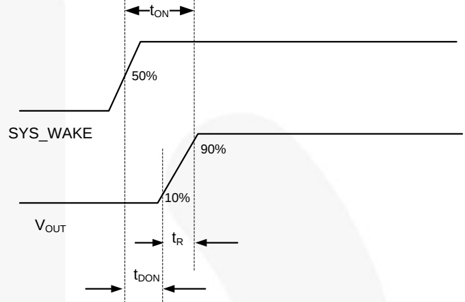
图 29. 时序图 (SYS_WAKE 与 V OUT 的关系)
