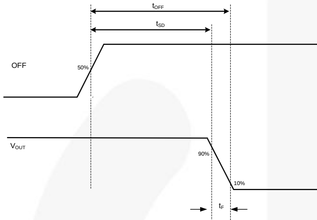
图 28. 时序图 (OFF 与 V OUT 的关系)
