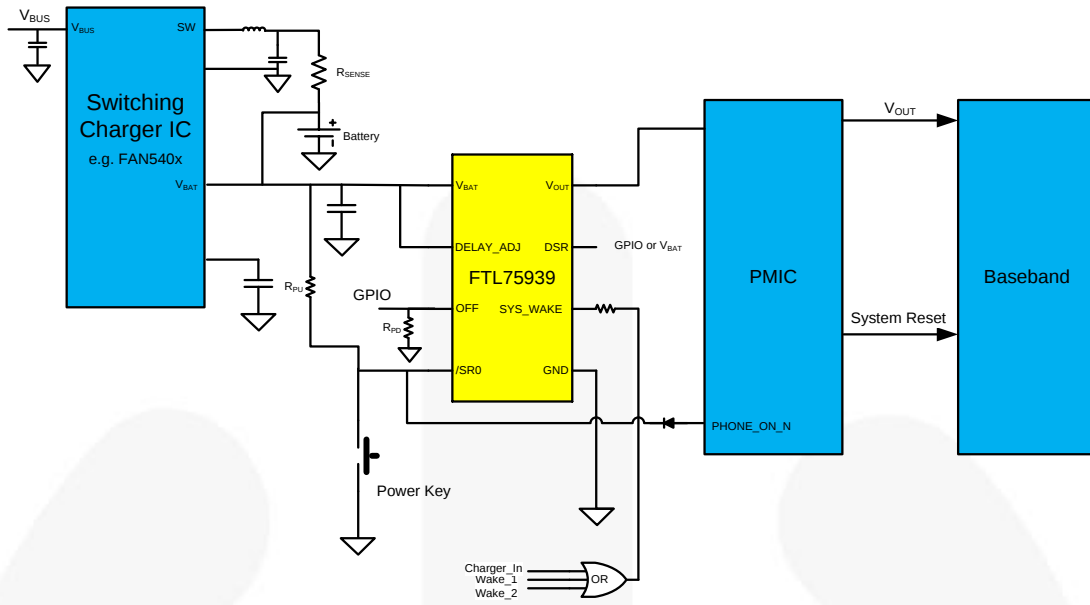
图 1. 带独立开关充电器IC的典型应用
