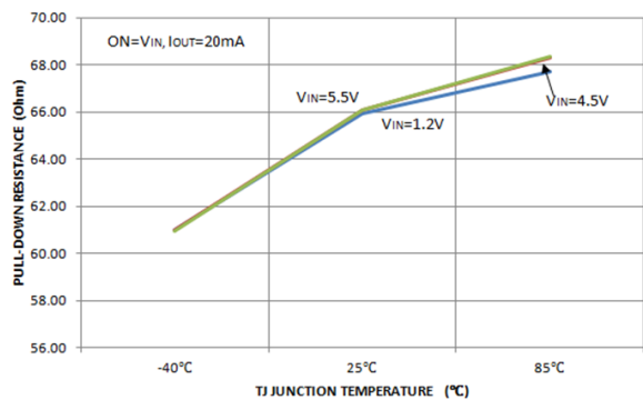
图 14. 输出放电电阻 R_{PD} 与温度的关系
