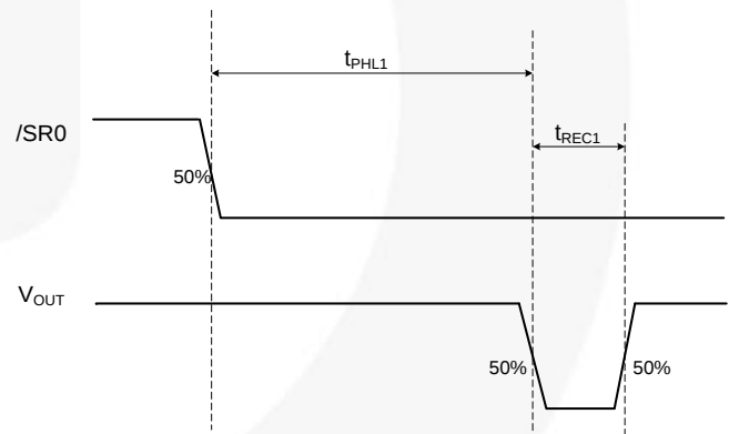
图 31. 复位计时
