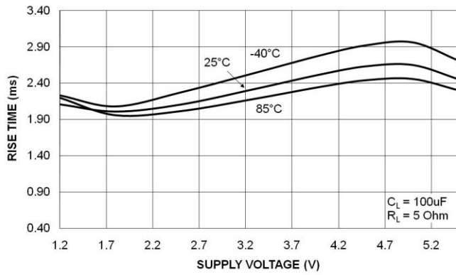
图 22. t_R 与电源电压的关系
