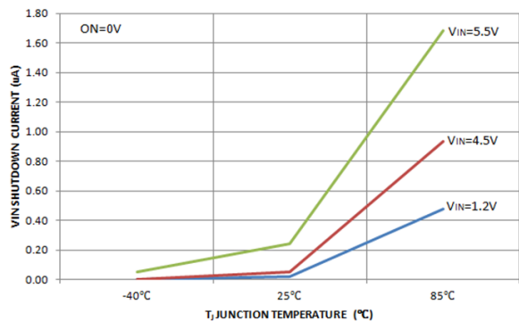
图 6. 关断电流与温度的关系
