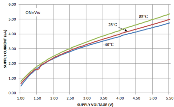
图 11. 静态电流与电源电压的关系
