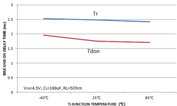
图 20. t_r/t_{DON} 与温度的关系
