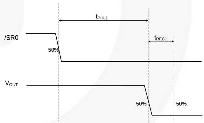
图 31. 复位计时
