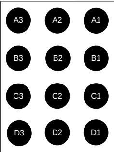
图 5. 底视图
