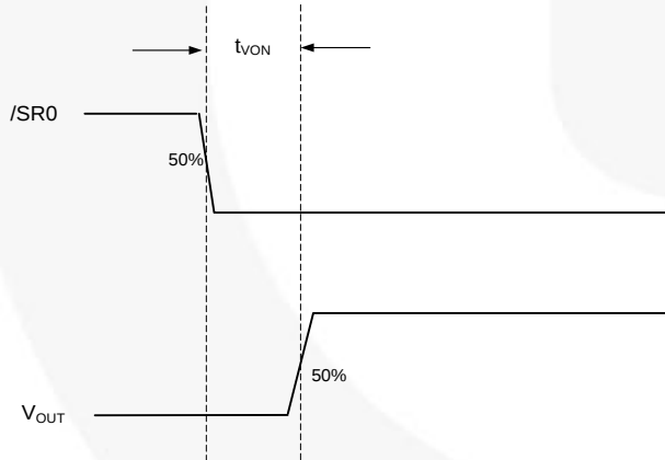
图 30. /SR0 上电
