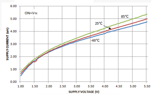
图 11. 静态电流与电源电压的关系
