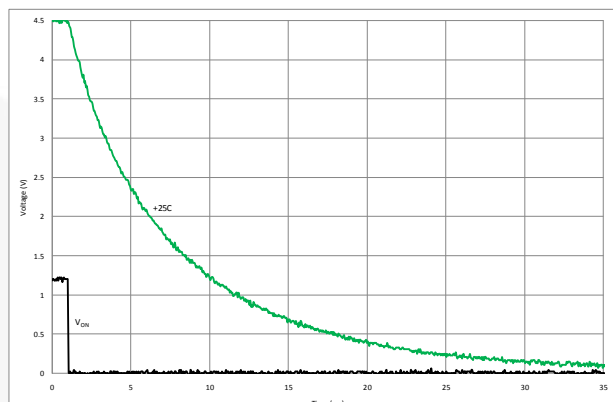
图 23. 关断响应 ( V_{BAT}=4.5V , C_{IN}=10\mu F , C_L=100\mu F , 无外部 R_L )
