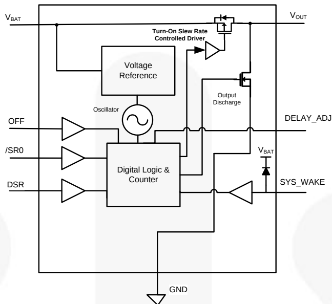
图 3. 框图
