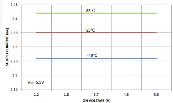
图 13. 静态电流与导通电压的关系 (V BAT =5.5 V)
