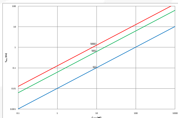
图 27. 下降时间与外部容性负载的关系 ( R_L=5\Omega 、 50\Omega 和 500\Omega )
