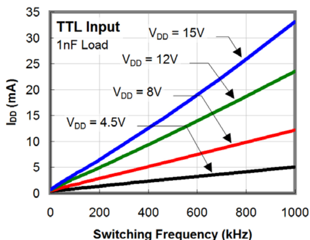
图 14. I_{DD} (1 nF 负载) 与频率的关系
