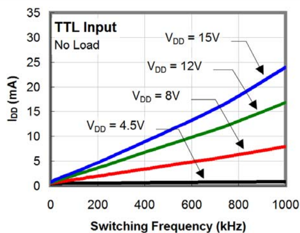
图 12. I_{DD} (无负载) 与频率的关系
