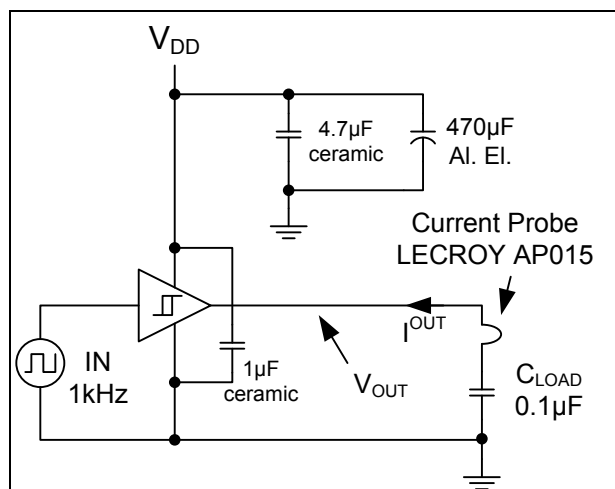
图 41. 准静态 I_{\text{OUT}}/V_{\text{OUT}} 测试电路
