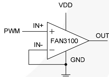
图 45. 使能的双输入驱动器, 同相配置
