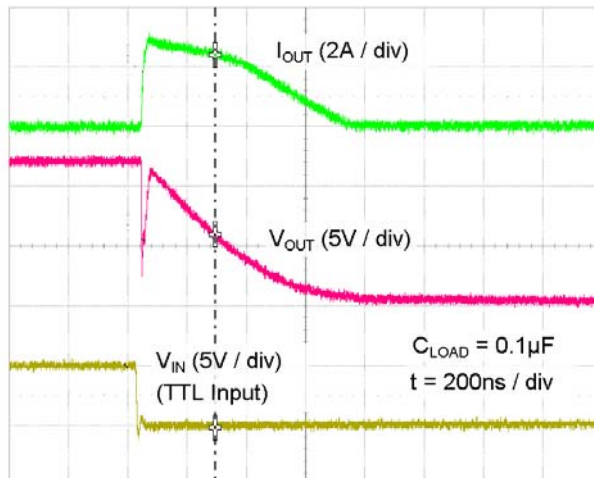
图 38. V_{\text{DD}}=12\text{ V} 时的准静态灌电流波形
