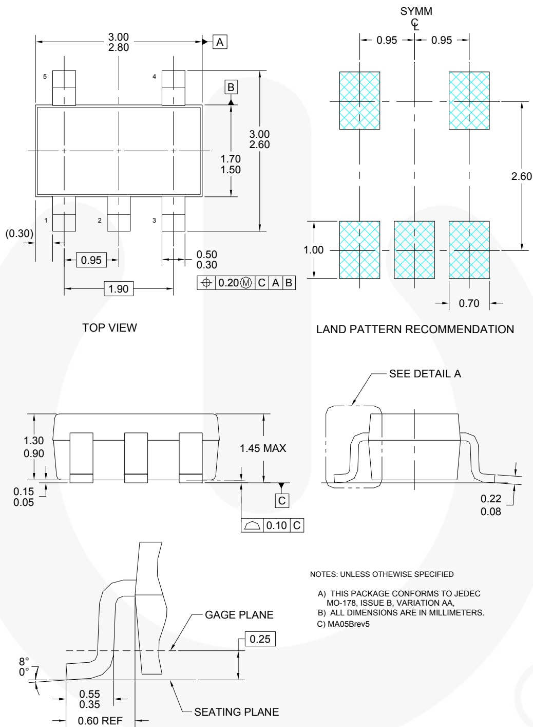
图 54. 5 引脚 SOT-23
