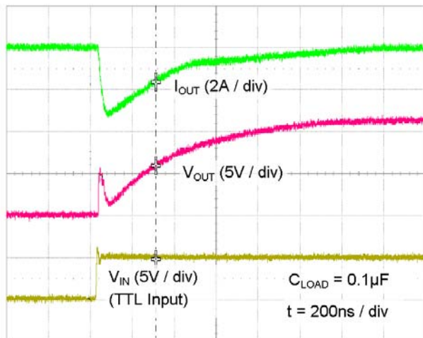
图 37. V_{\text{DD}}=12\text{ V} 时的准静态源电流波形
