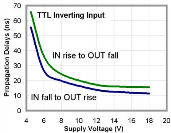
图 25. 传播延迟与电源电压
