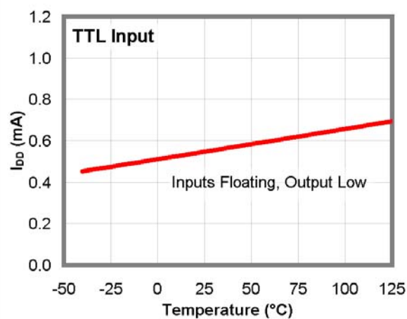
图 16. I_{DD} (静态) 与温度的关系
