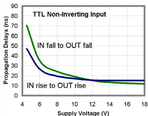
图 27. 传播延迟与电源电压
