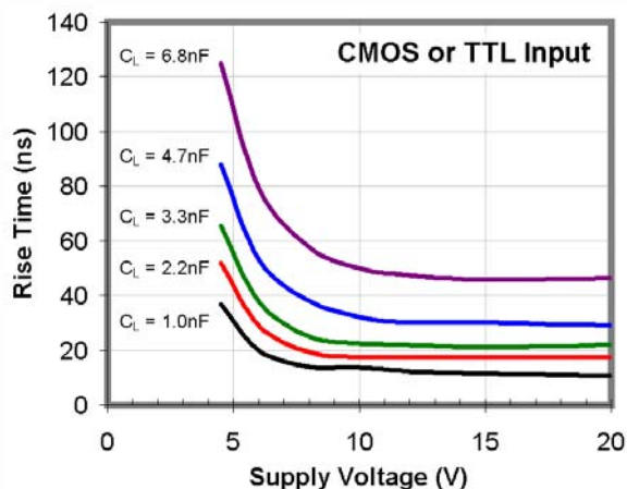
图 33. 上升时间与电源电压的关系
