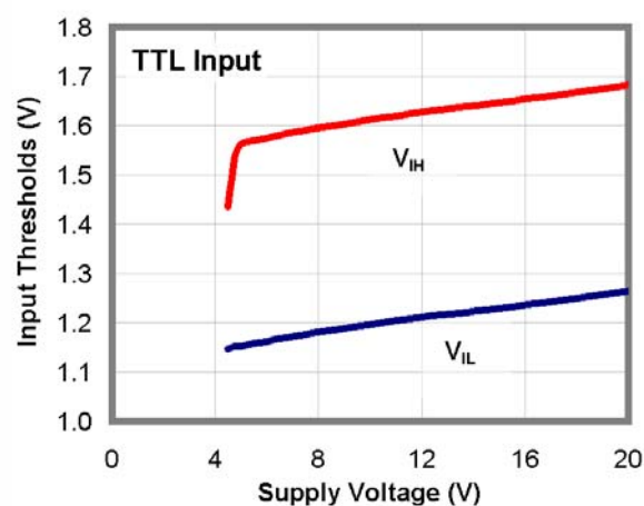
图 18. 输入阈值与电源电压的关系
