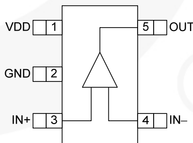
图 2. SOT23-5 (俯视图)
