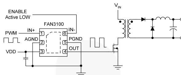
图 49. 正向转换器，初级端栅极驱动（如 MLP 封装所示）
