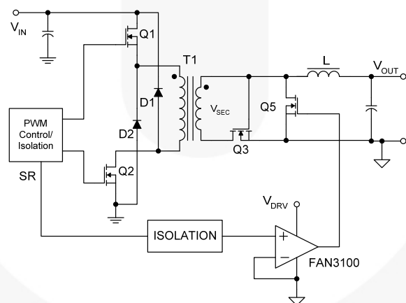
图 51. 次级同步整流驱动器
