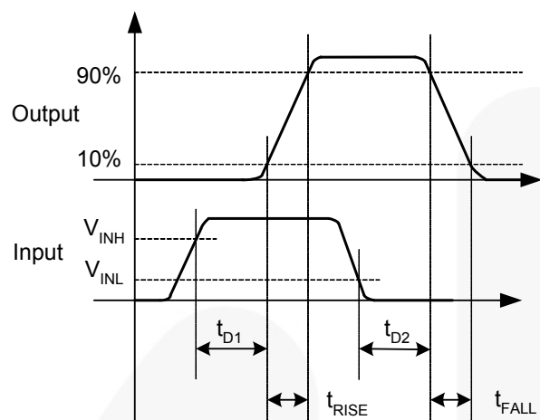
图 7. 同相
