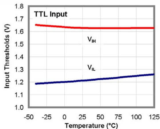
图 21. TTL 输入阈值与温度的关系
