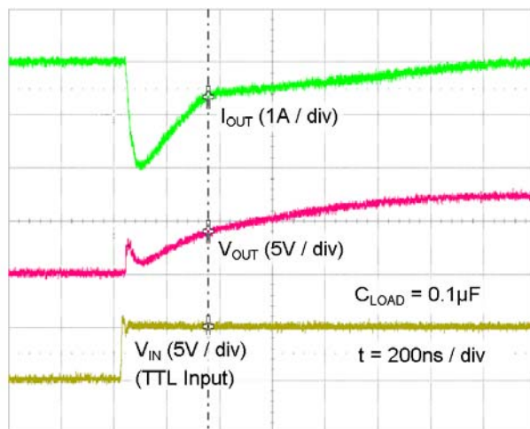
图 39. V_{\text{DD}}=8\text{ V} 时的准静态源电流波形
