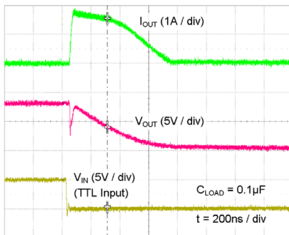
图 40. V_{\text{DD}}=8\text{ V} 时的准静态灌电流波形
