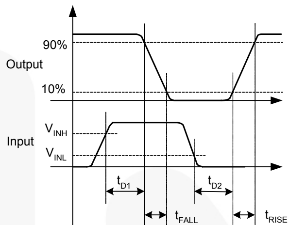
图 8. 反相
