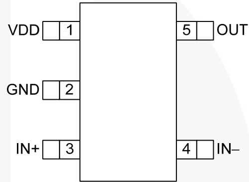
图 4. SOT23-5（俯视图）
