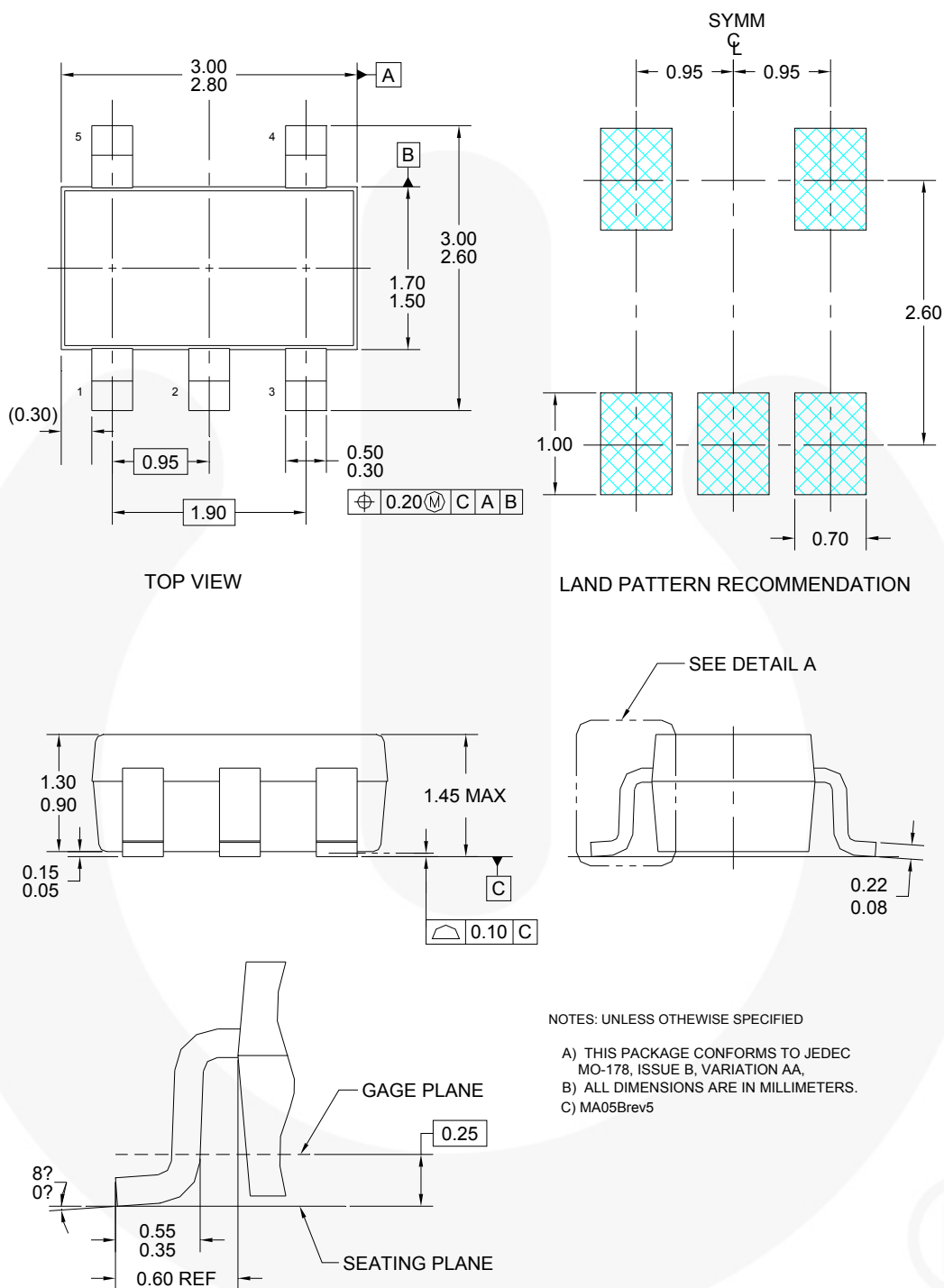
图 37. 5 引线 SOT-23
