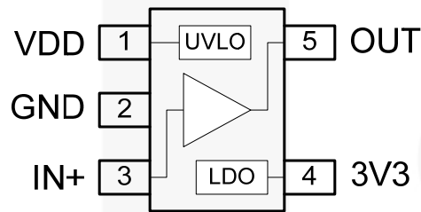
图 2. 俯视图
