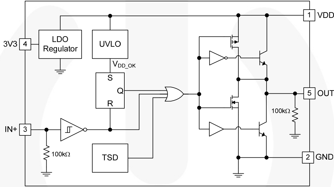
图 3. 简化框图
