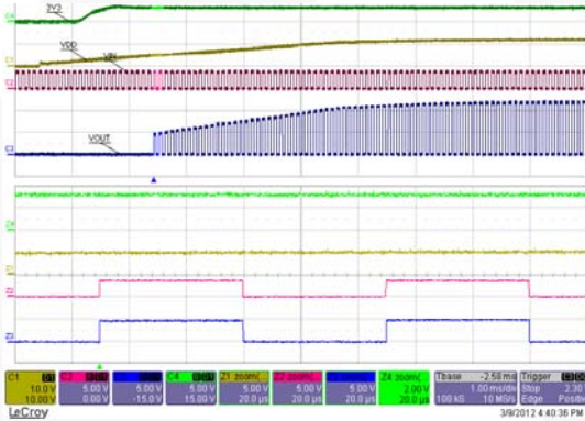
图 28. 3V3, V_{DD} > UVLO_{ON} 前
