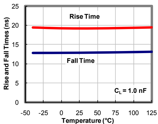
图 17. 上升和下降时间 vs. 温度
