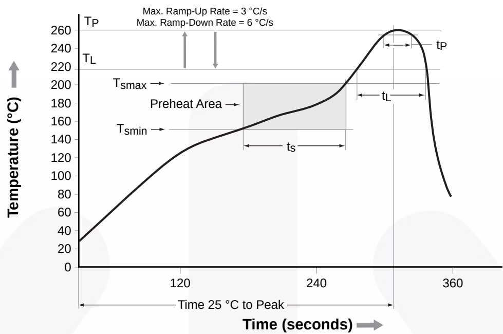
图 59. 回流焊数据
