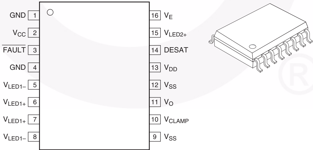
图 1. 引脚配置
