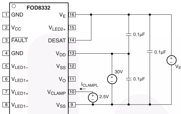
图 42. 钳位低电平灌电流 ( I_{CLAMPL} ) 测试电路
