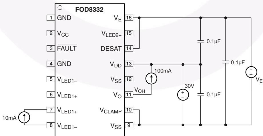
图 35. 高电平输出电压 ( I_{OH} ) 测试电路
