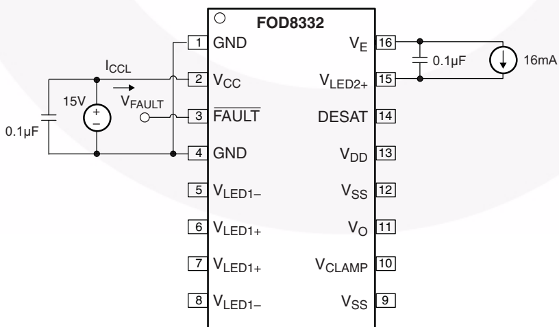
图 44. 故障低电平电源电流 ( I_{CCL} ) 测试电路
