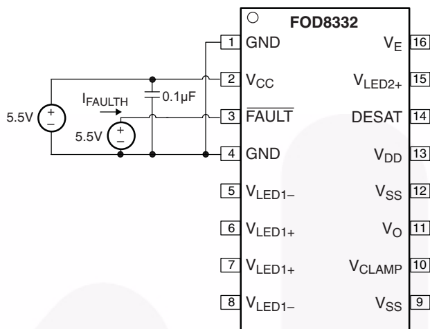
图 45. 故障高电平输出电流 ( I_{FAULTH} ) 测试电路
