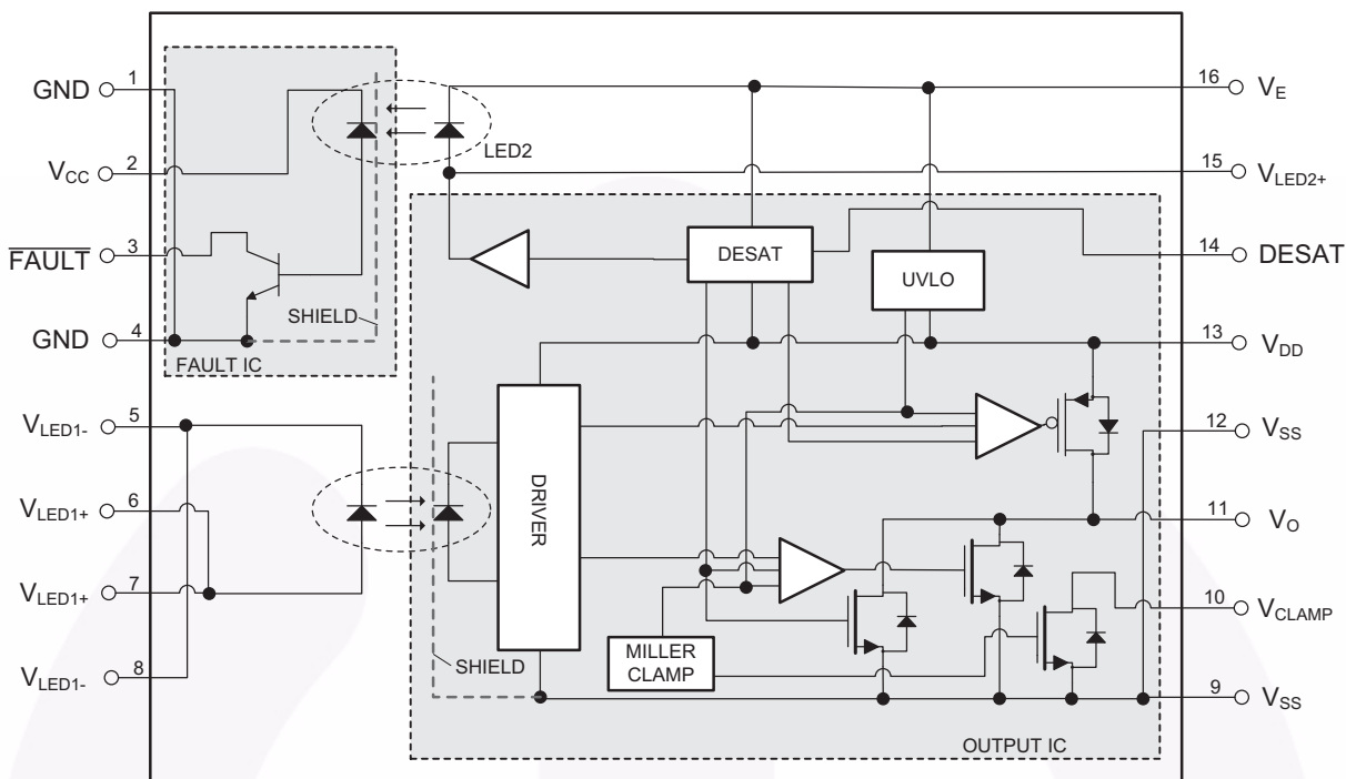
框图
