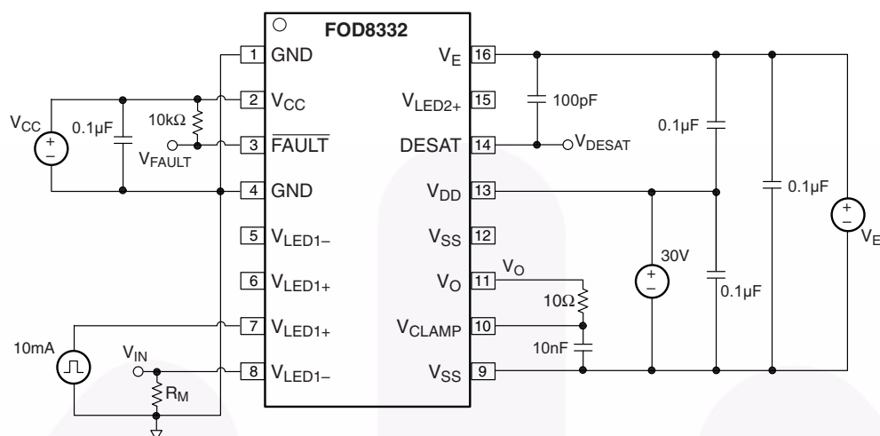
图 48. DESAT 检测延迟 ( t_{\text{DESAT}(90\%)} )、 t_{\text{DESAT}(10\%)} 、 t_{\text{DESAT}(\text{LOW})} 、DESAT 检测到低电平故障信号延迟 ( t_{\text{DESAT}(\text{FAULT})} )、重置为高电平故障信号延迟 ( t_{\text{RESET}(\text{FAULT})} )、DESAT 输入静音 ( t_{\text{DESAT}(\text{MUTE})} ) 测试电路
