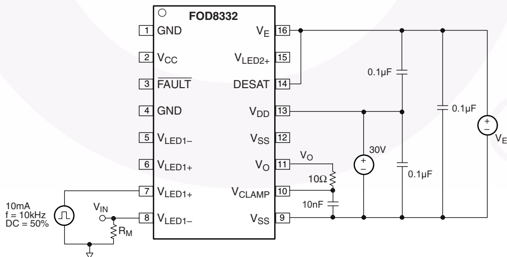
图 47. 传播延迟 ( t_{PLH} 、 t_{PHL} )、上升时间 ( t_R )、下降时间 ( t_F )、脉冲宽度失真度 (PWD) 测试电路
