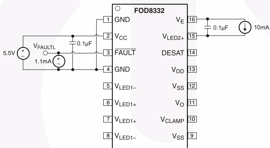
图 46. 故障低电平输出电压 ( V_{FAULTL} ) 测试电路
