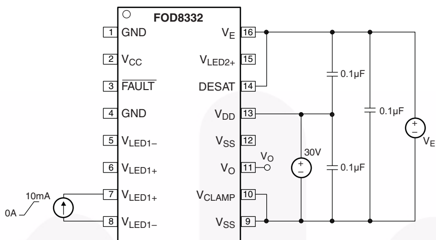
图 30. 阈值输入电流低电平至高电平 ( I_{FIH} ) 测试电路
