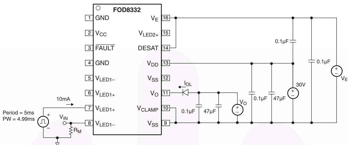
图 33. 低电平输出电流 ( I_{OL} ) 测试电路
