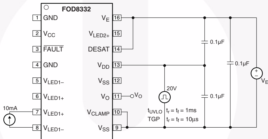
图 49. 欠压锁定延迟 ( t_{\text{UVLO}} )、供电时间 ( t_{\text{GP}} ) 测试电路
