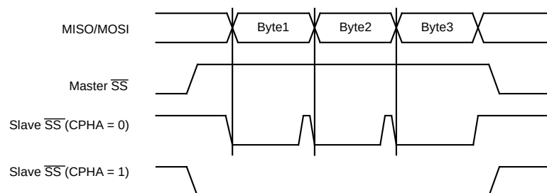
CPHA/SS时序
